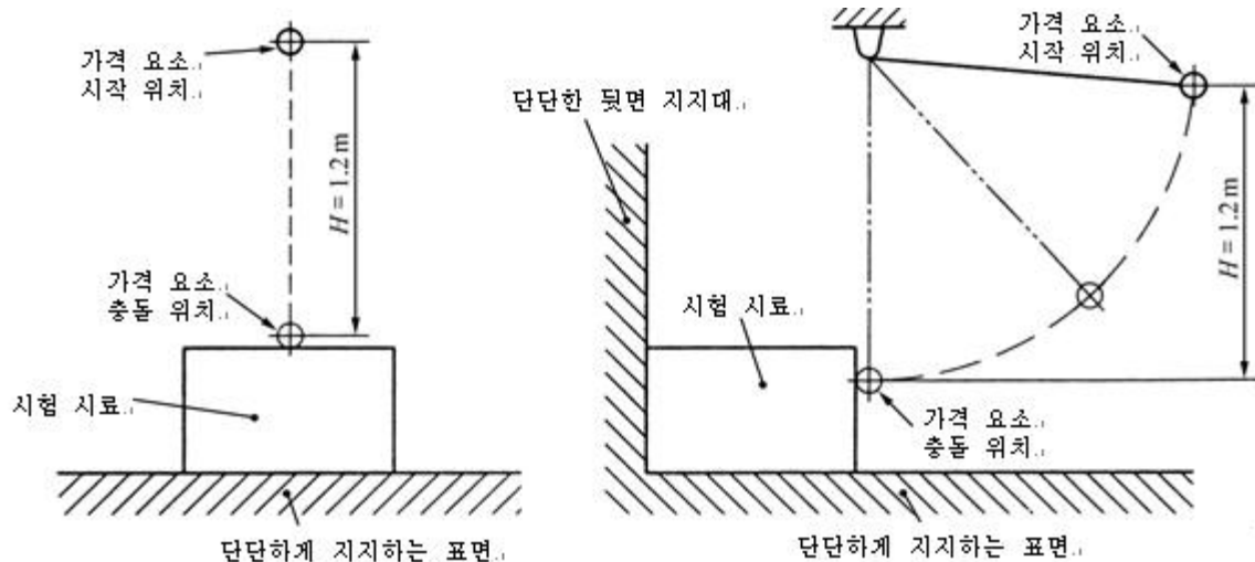
그림 1 가격 요소를 이용한 충돌 시험
