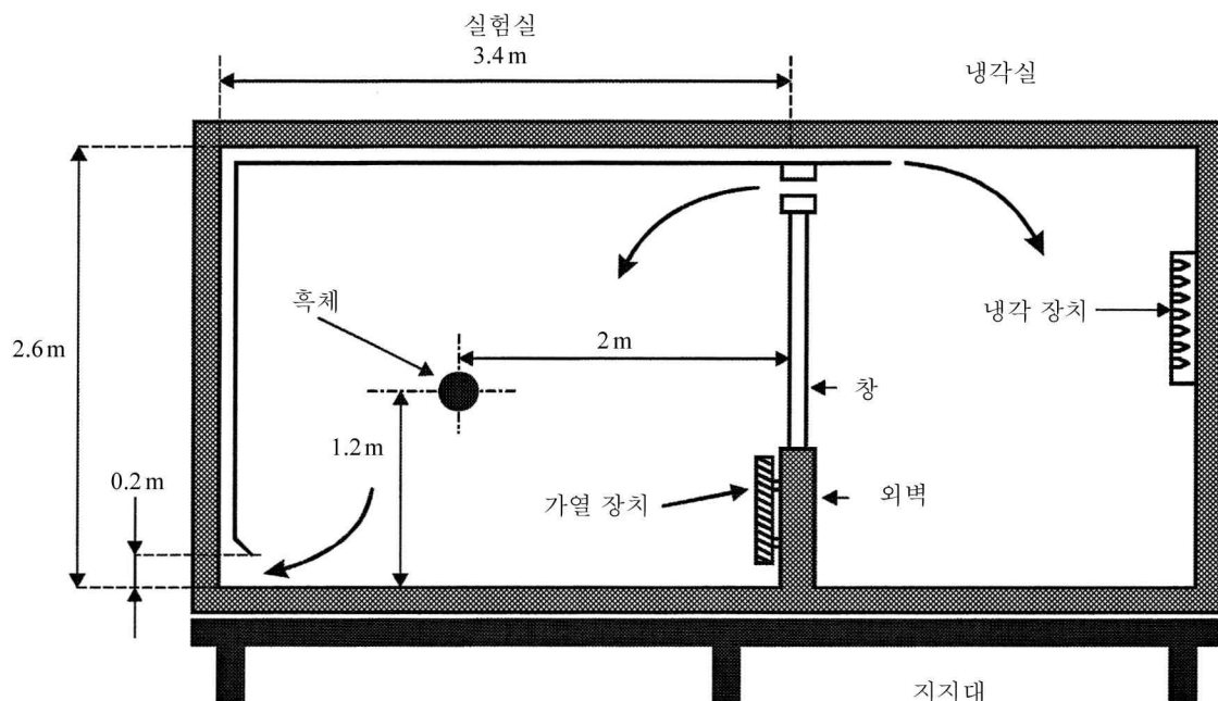
그림 B.1 환경 시험실의 예
