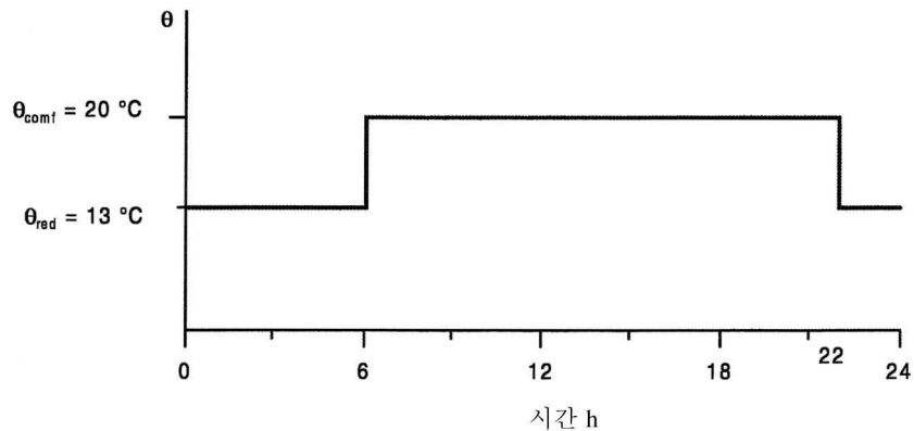
그림 C.1 안락한 실내 온도의 예
