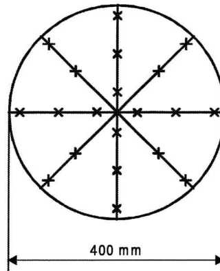
그림 A.3 공기 배출구 내의 열전대 배치
