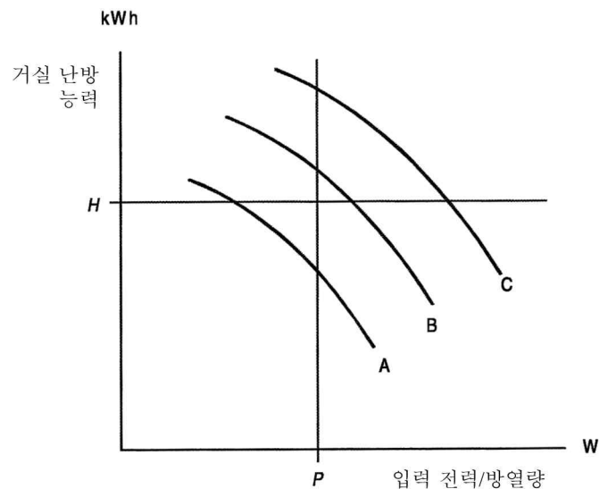
그림 C.9 다른 축열식 난방기들의 적합성에 대한 예
