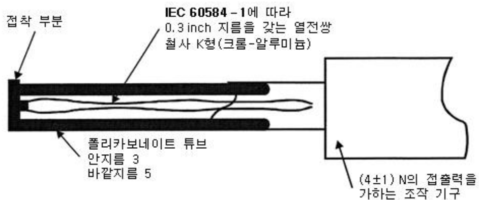
그림 4 표면 온도를 측정하기 위한 프로브
