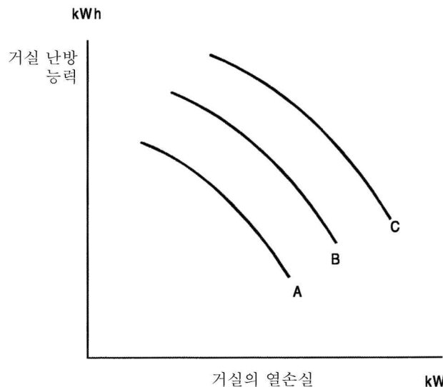
그림 C.4 기타 축열식 난방기에 대한 실내 난방 용량
