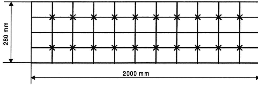
그림 A.2 공기 인입구 내의 열전대 배치
