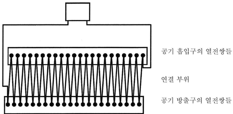
그림 A.4 열전대의 접속
