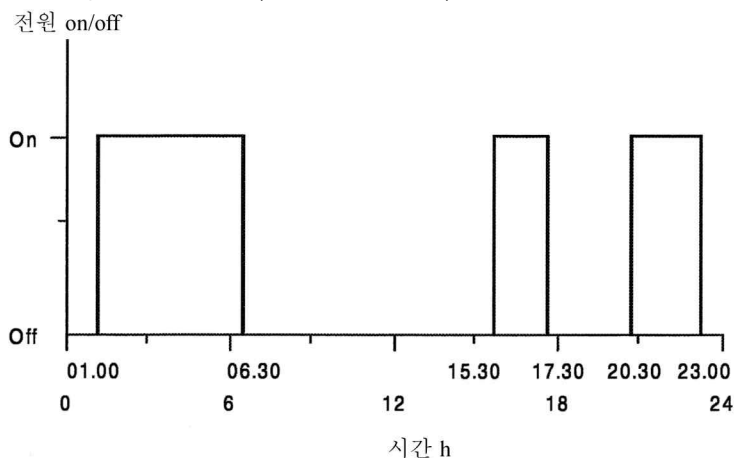
그림 C.2 일일 축열 계획의 예
