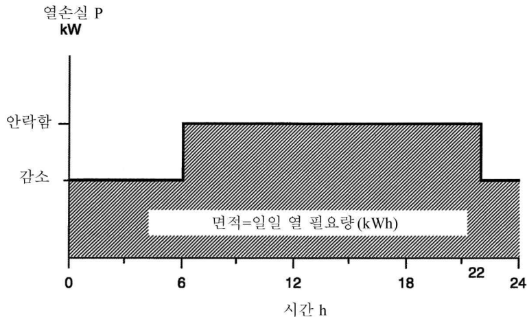
그림 C.5 열손실의 예
