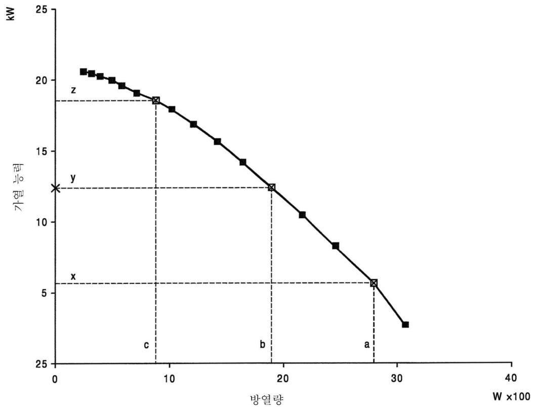
그림 3 실내 난방 용량
