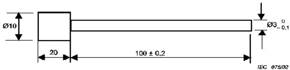
그림 101 은폐 잠금장치에 대한 시험막대
