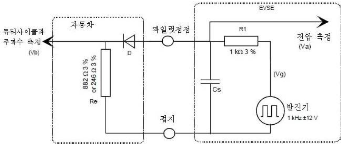
그림 A.2 - 간이 제어 파일럿 회로
