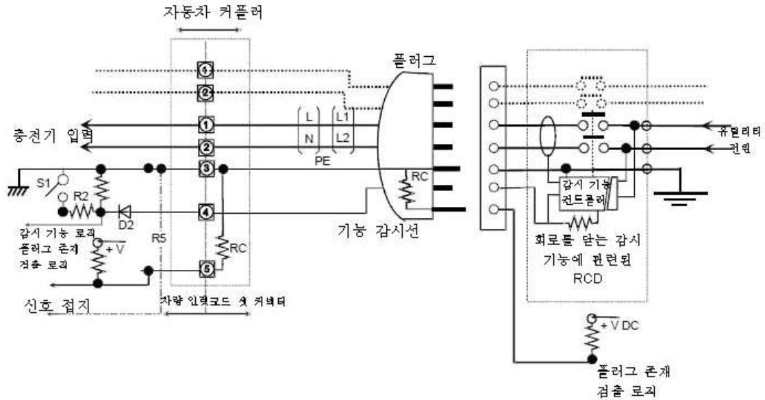
그림 B.5 - 근접 푸시버튼 스위치 S3이 없는 기본 단상 자동차 커플러를 사용한 모드 3의 B형
