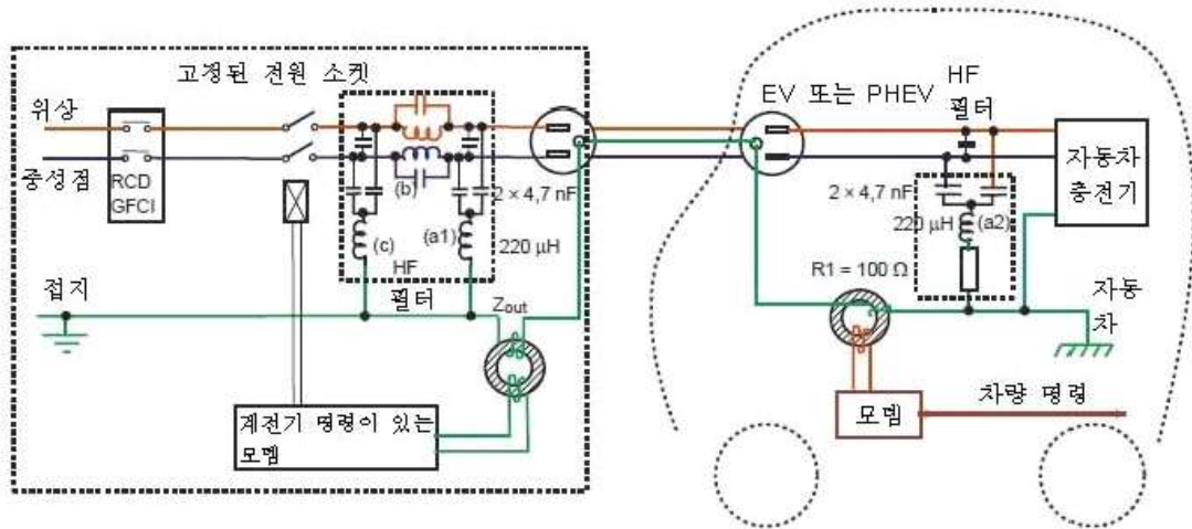
그림 C.1 - 보조선이 없는 파일럿 기능의 예
